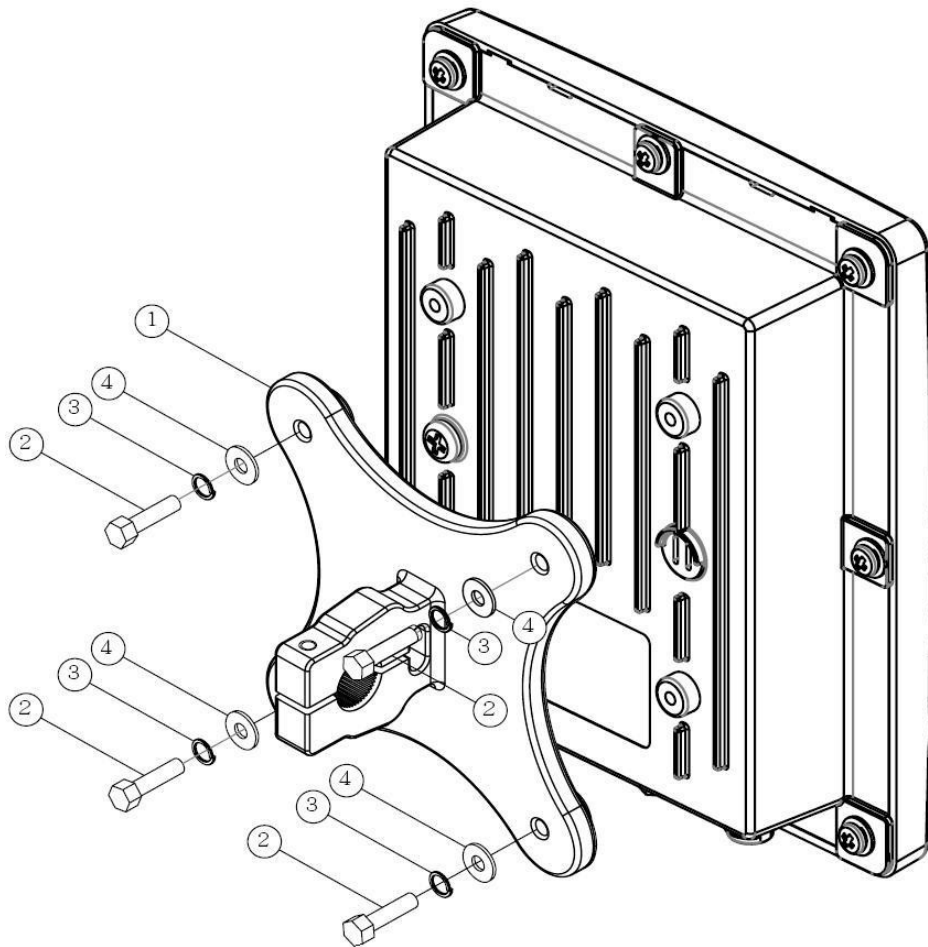
Abbildung 7 Montage des Grundrahmens – Diagramm I
