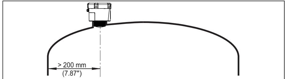
Abb. 5: Montage des Radarsensors an runden Behälterdecken
