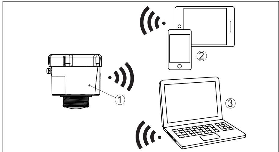
Abb. 3: Drahtlose Verbindung zu Standard-Bediengeräten über Bluetooth
