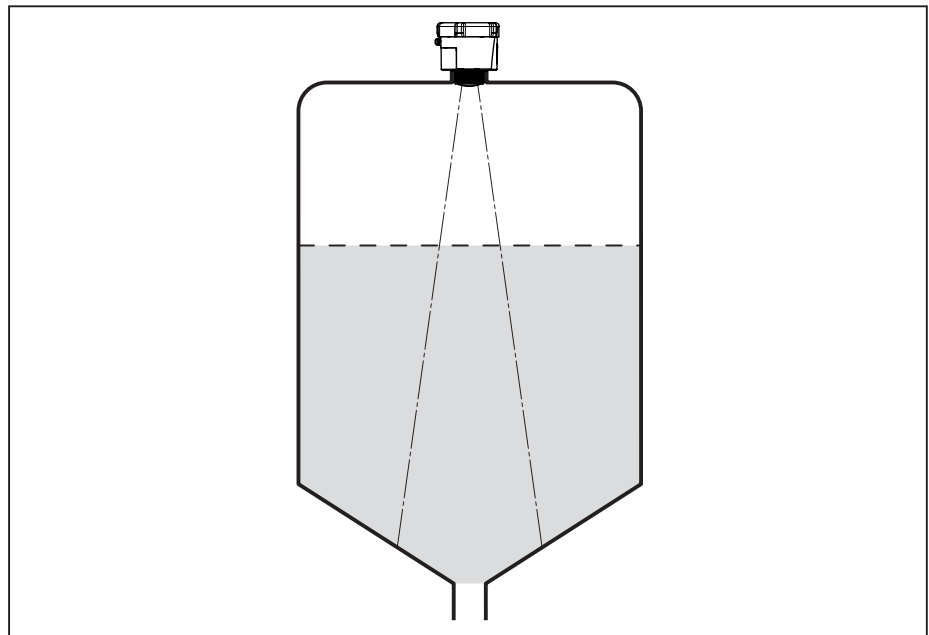
Abb. 6: Montage des Radarsensors an Behältern mit konischem Boden
