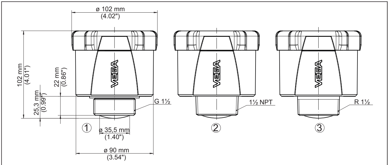
Abb. 29: Maße VEGAPULS Air 41
