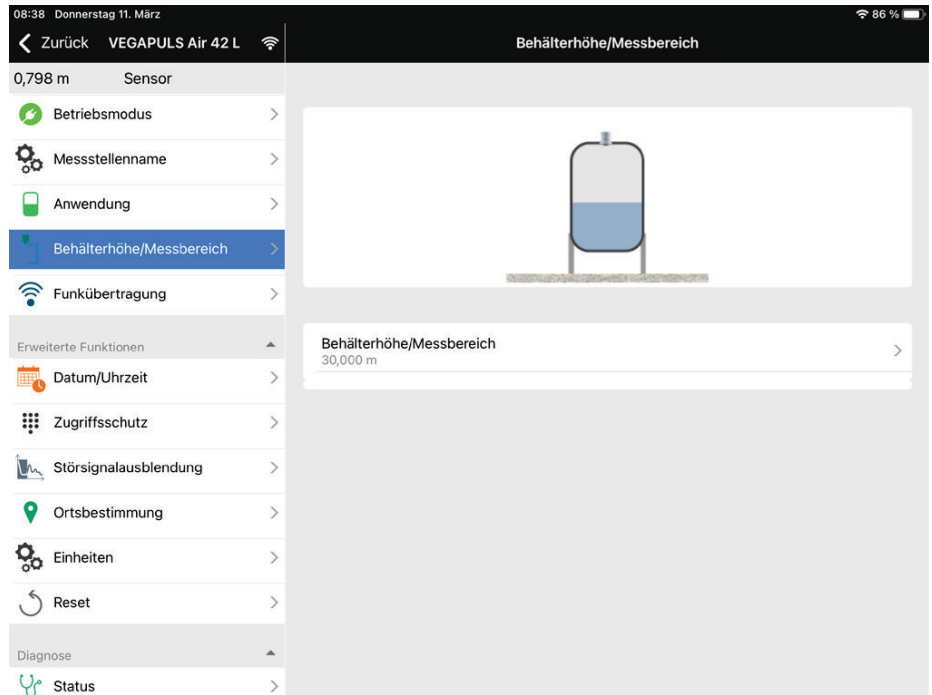
Abb. 21: Beispiel einer App-Ansicht - Menüpunkt Behälterhöhe, Messbereich
