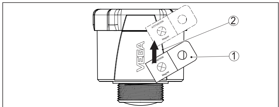
Abb. 14: Sensor aktivieren per Magnet
