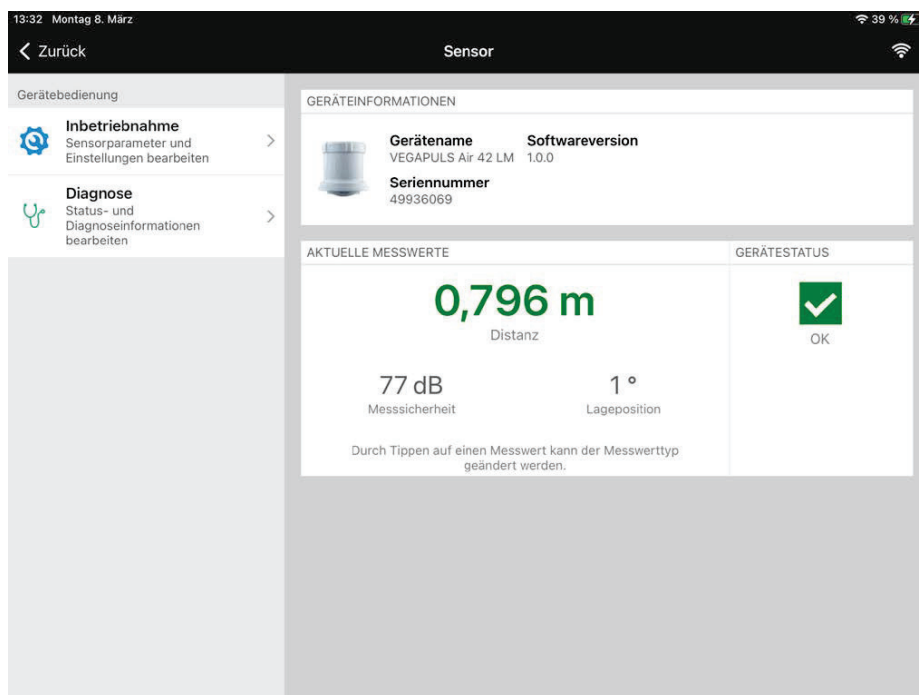
Abb. 20: Beispiel einer App-Ansicht - Geräteinformationen, Messwerte
