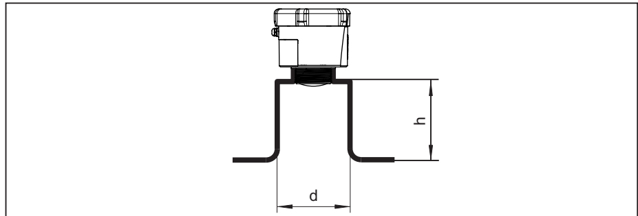
Abb. 9: Rohrstützenmontage bei abweichenden Rohrstützenmaßen
