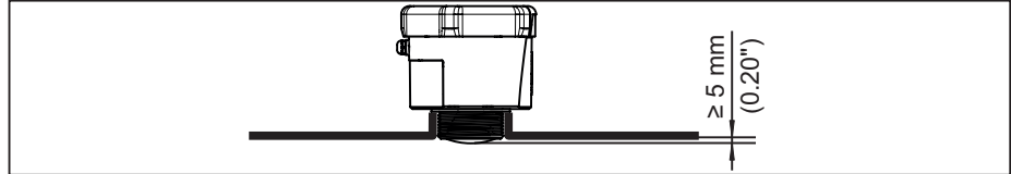
Abb. 8: Empfehlenswerte Rohrstützenmontage des VEGAPULS Air 41
