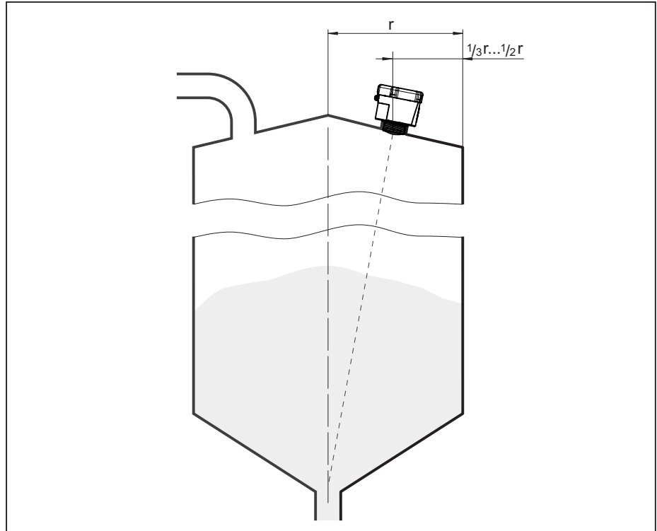
Abb. 11: Montageposition und Ausrichtung
