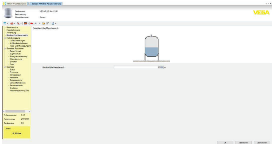
Abb. 23: Beispiel einer DTM-Ansicht - Menüpunkt Behälterhöhe, Messbereich
