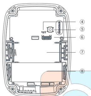
Innenansicht: ④ LED ⑤ Ein-/Aus-Taste ⑥ USB Typ. C ⑦ Erweiterbarer Akkufach ⑧ Akku
