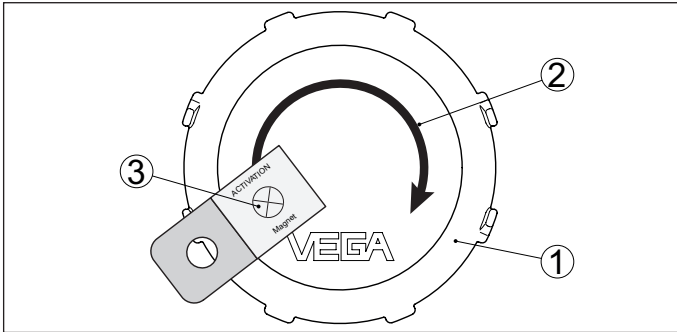
Abb. 20: Sensor aktivieren - Magnet
