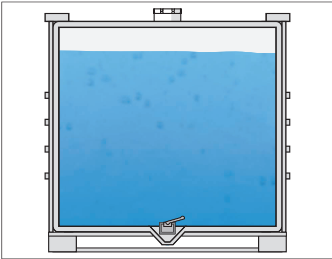
Abb. 12: Füllstandmessung mit VEGAPULS Air 23 im IBC-Behälter
