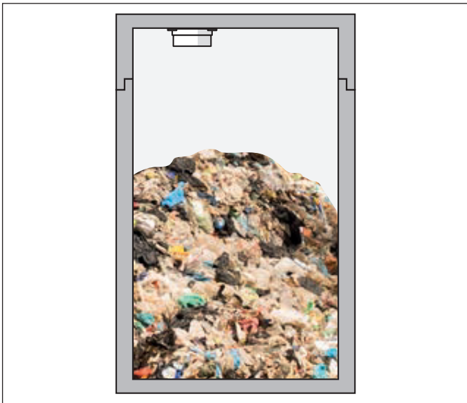
Abb. 13: Füllstandmessung mit VEGAPULS Air 23 im Abfallbehälter
