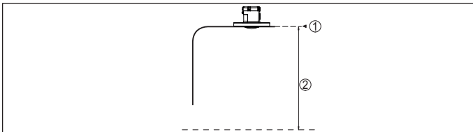
Abb. 2: Daten zur Eingangsgröße VEGAPULS Air 42
