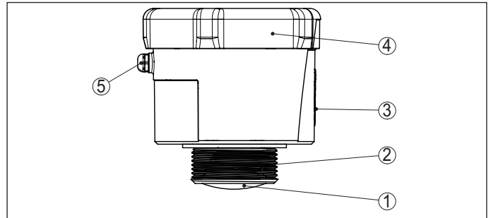
Abb. 6: Komponenten des Radarsensors VEGAPULS Air 41 (Beispiel Ausführung mit Gewinde G1½)
